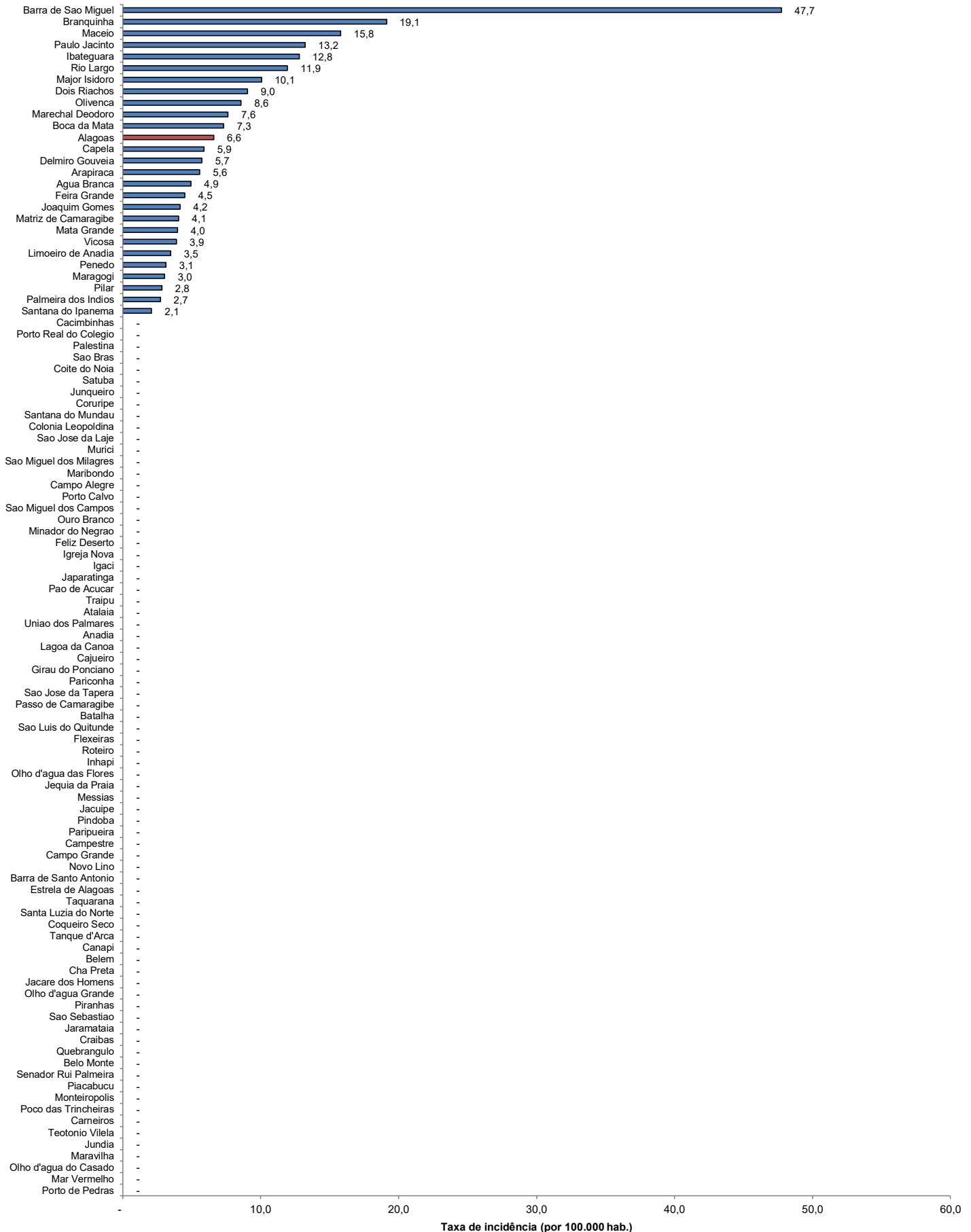
Gráfico 14 – Taxa de incidência (por 100.000 hab.) da COVID-19, nos últimos 28 dias (10 de dezembro a 05 de janeiro), segundo município de residência. Alagoas, 2021 e 2022.
