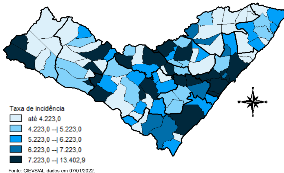
Figura 4 – Taxa de incidência (por 100.000 hab.) dos casos confirmados da COVID-19, nos últimos 28 dias (10 de dezembro a 06 de Janeiro), segundo município de residência. Alagoas, 2021 e 2022.
