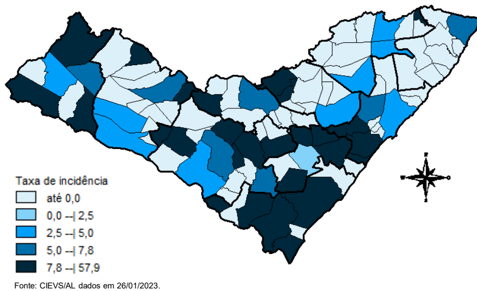
Figura 4 – Taxa de incidência (por 100.000 hab.) dos casos confirmados da COVID-19, nos últimos 28 dias (29 de dezembro/22 a 25 de janeiro/23), segundo município de residência. Alagoas, 2023.
