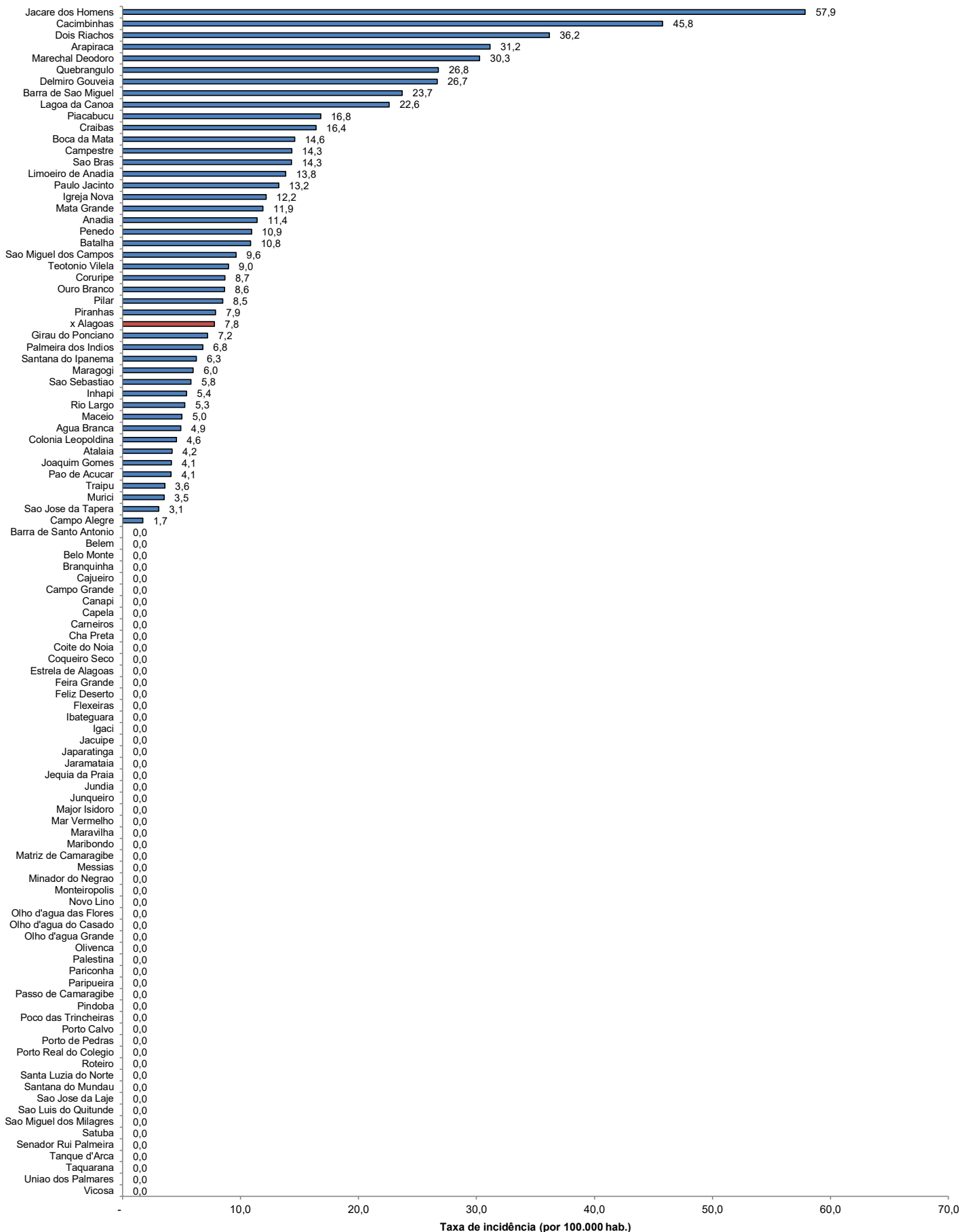
Gráfico 14 – Taxa de incidência (por 100.000 hab.) da COVID-19, nos últimos 28 dias (29 de dezembro/22 a 25 de janeiro/23), segundo município de residência. Alagoas, 2023.
