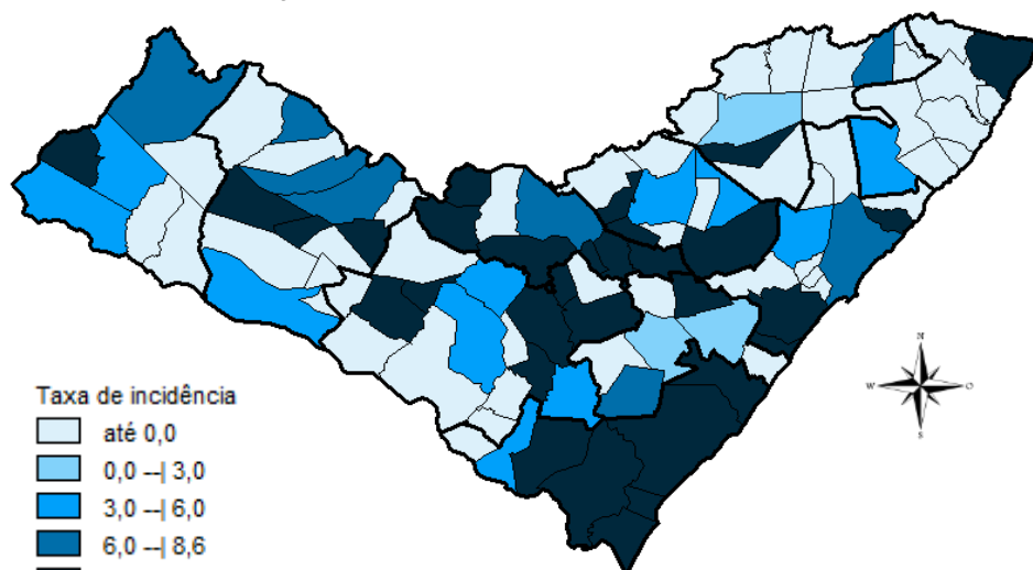
Figura 4 – Taxa de incidência (por 100.000 hab.) dos casos confirmados da COVID-19, nos últimos 28 dias (13 de janeiro a 09 de fevereiro), segundo município de residência. Alagoas, 2023.
